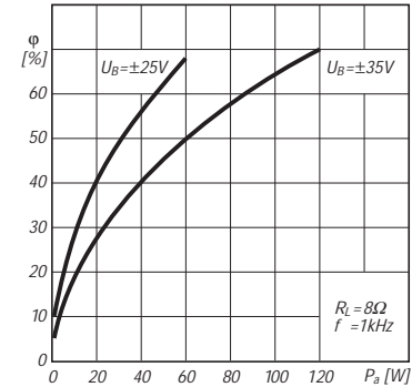
Bild 8: Der Wirkungsgrad steigt mit der Endstufen-Ausgangsleistung.
