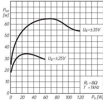
Bild 7: Verlustleistung als Funktion der Endstufen-Ausgangsleistung
