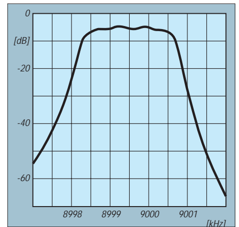
Bild 8: Eine Simulation mit willkürlich veränderten Bauteilwerten gibt Aufschluß über die statthaftern Toleranzen.
