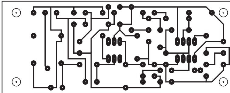
Bild 3: Platinenlayout
