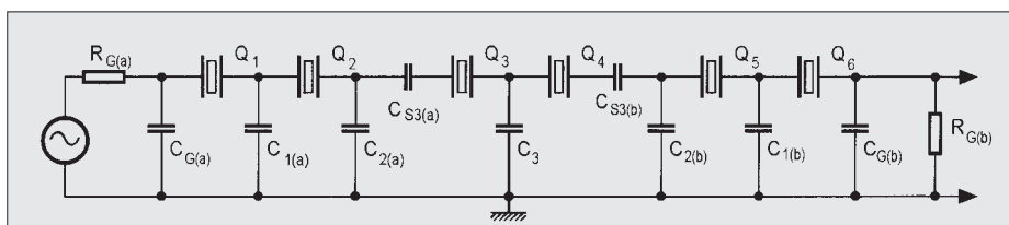
Bild 5: Ausgehend von dieser Grundschaltung wurden, nach Berechnung der Bauteilwerte, Simulations- und Wobbelprogramme erstellt.
