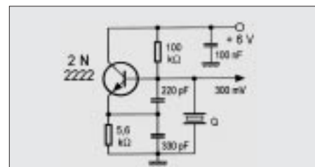
Bild 4: Mit diesem Oszillator kann man Quarze betreffs Frequenz und Dämpfung vergleichen.
