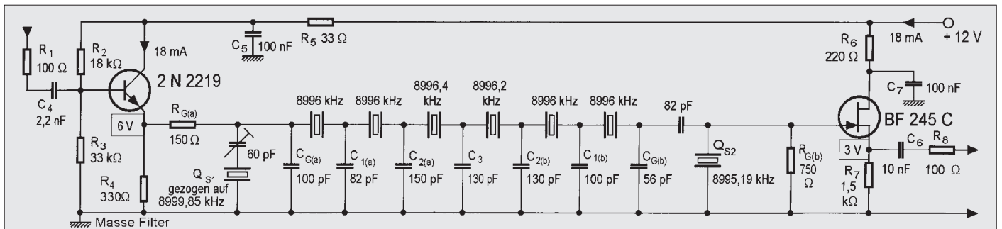
Bild 14: Steilere Filterflanken erhält man, indem man Q_{S1} und Q_{S2} etwas oberhalb und unterhalb des Durchlassbereiches in einer Ableitfunktion einsetzt.
