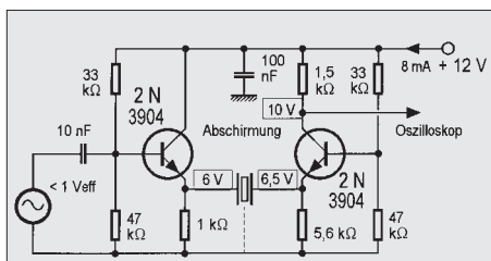
Bild 2: Schaltung zur direkten Bestimmung der Serien- und Parallelresonanzen von Quarzen.
