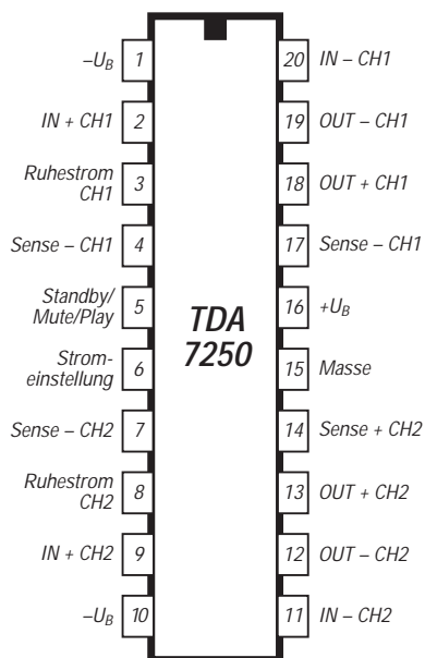
Bild 1: Pinbelegung
